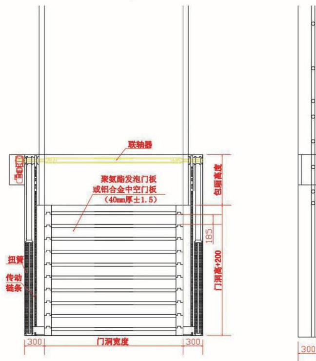
垂直硬质快卷门示意图
