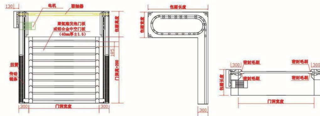
椭圆硬质快卷门示意图
