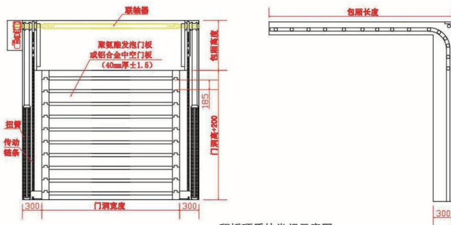
翻板硬质快卷门示意图
