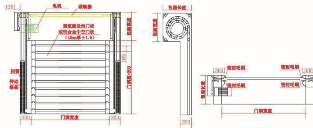
螺旋硬质快卷门示意图
