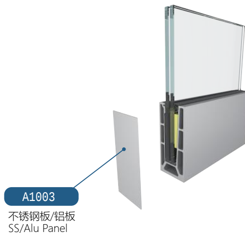
收口 End Cap
