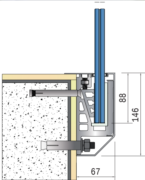
尺寸 Detail
