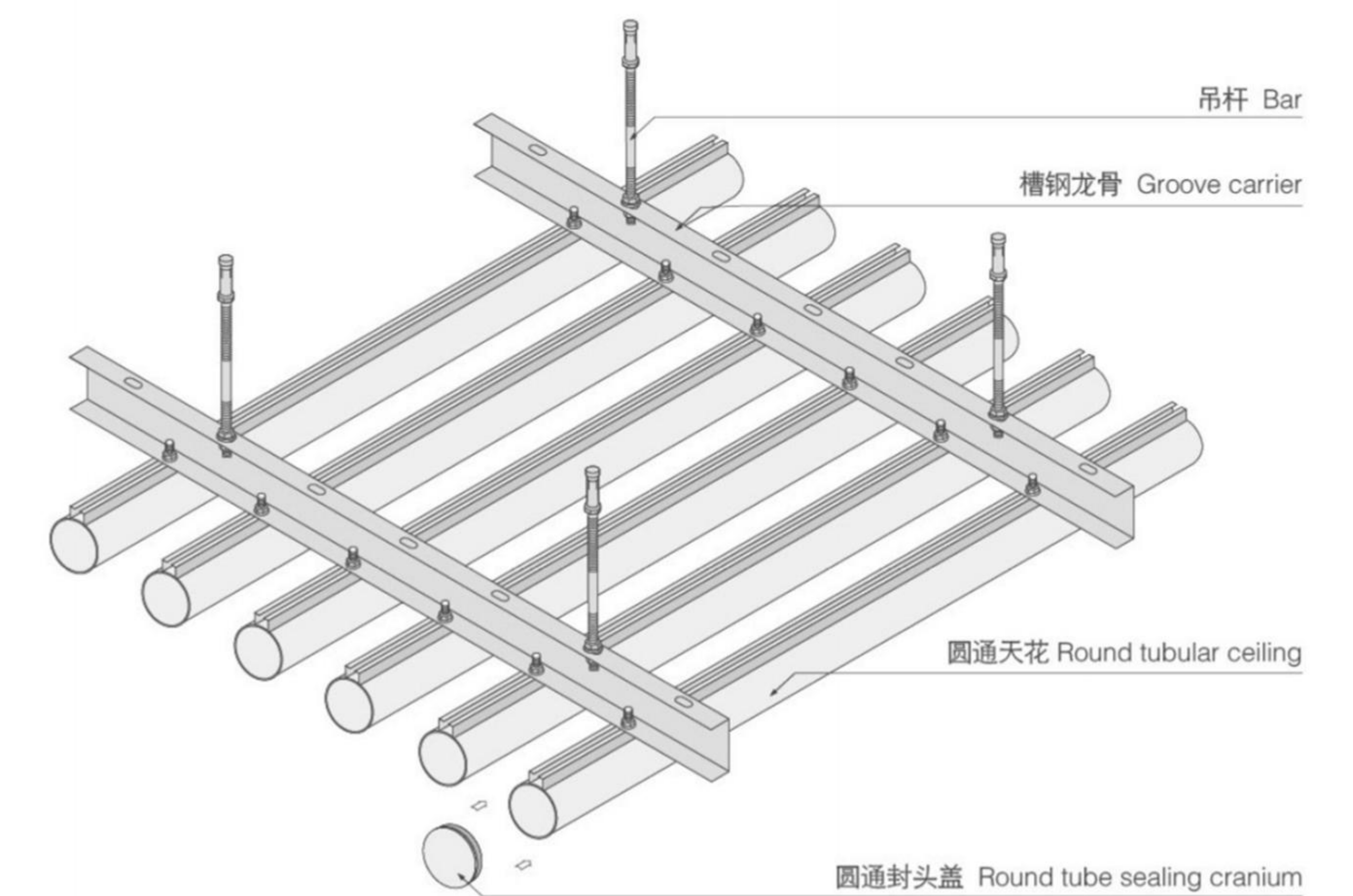
圆通安装示意图 ②
