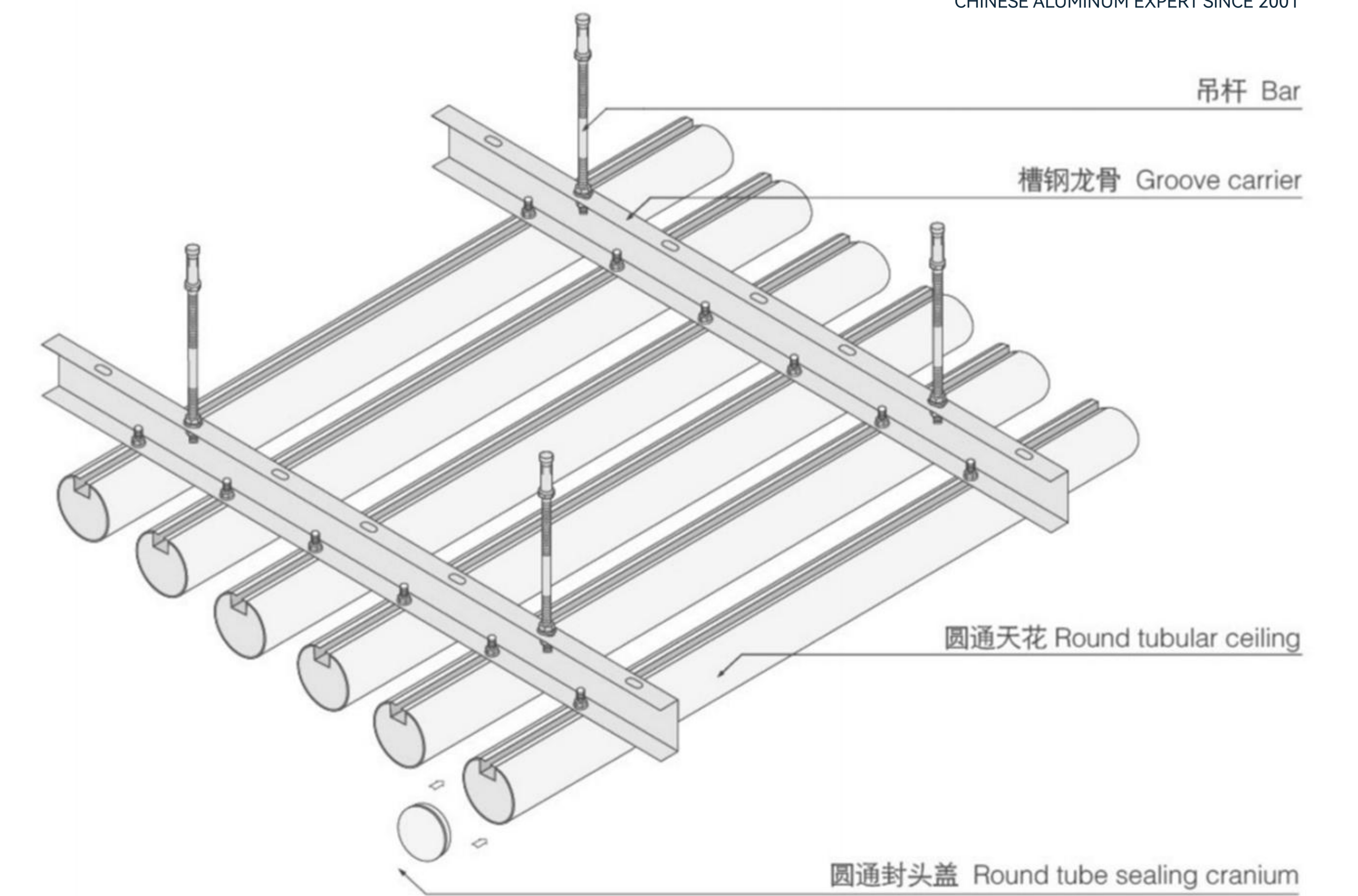
圆通安装示意图 ①
